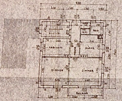
- OBERGESCHOSS -
