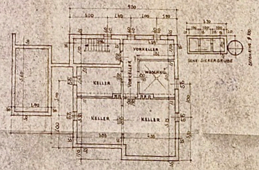
- KELLERGESCHOSS -
