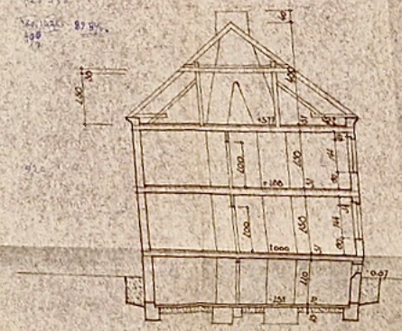
- SCHNITT -
