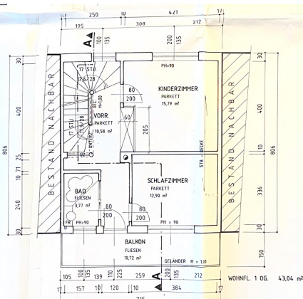
GRUNDRISS 1. OBERGESCHOSS
