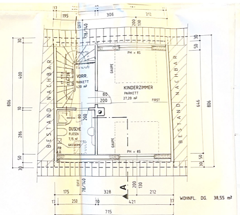
GRUNDRISS DACHGESCHOSS
